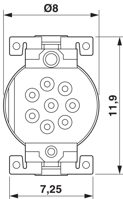
Rysunek wymiarowy
