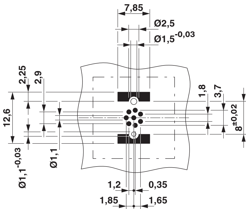
Otworowanie/geometria płytek lutowniczych
