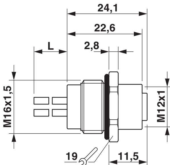
Rysunek wymiarowy
