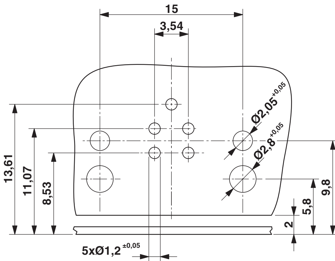
Schemat otworowania wyłącznie dla obudowy SACC-M12-SCO PLUG L90 (nr kat. 1436709)
