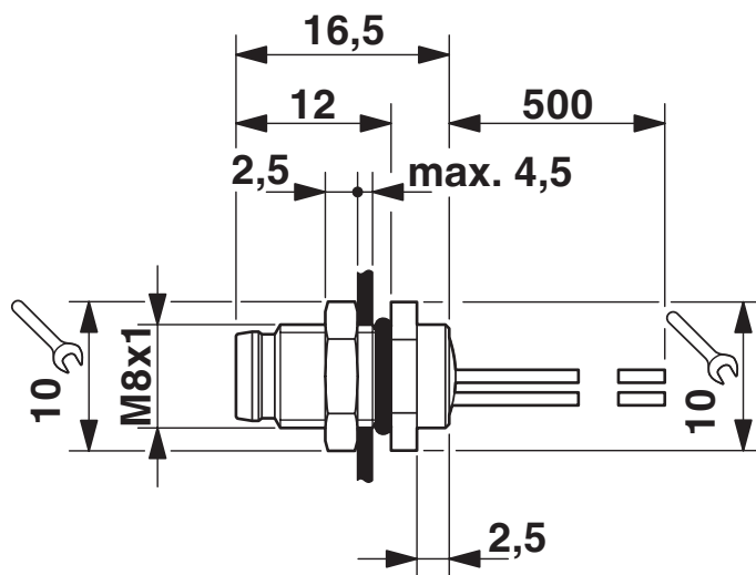
Rysunek wymiarowy
