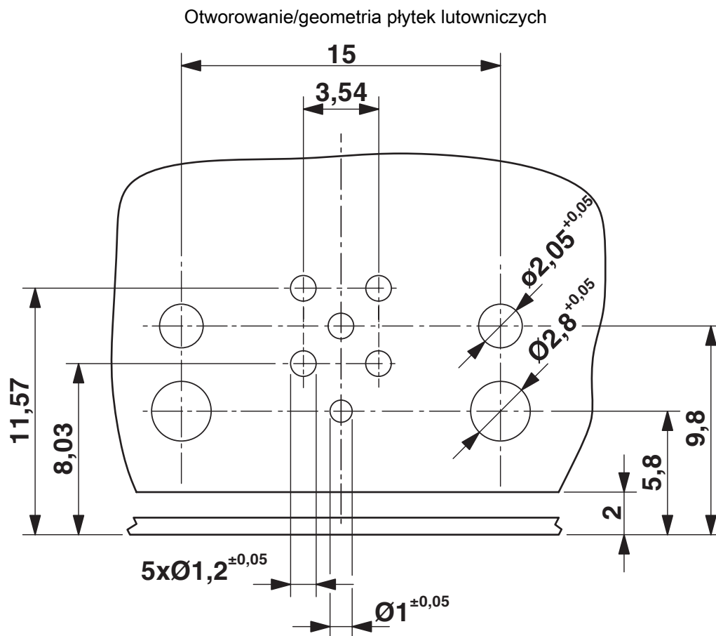
Rysunek wymiarowy
