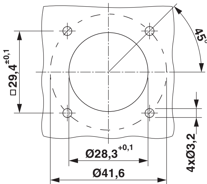
Rysunek wymiarowy
