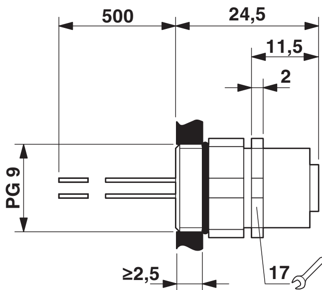
Rysunek wymiarowy
