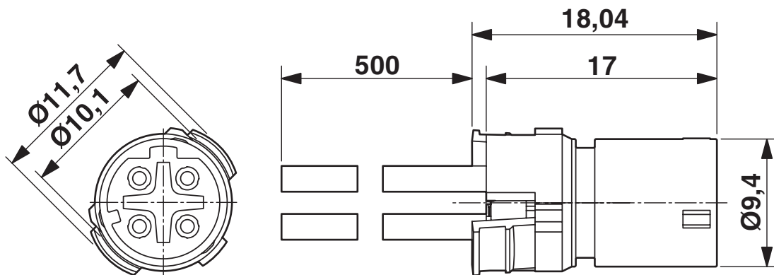
Rysunek wymiarowy
