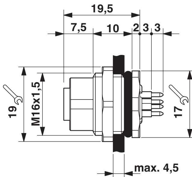
Rysunek wymiarowy
