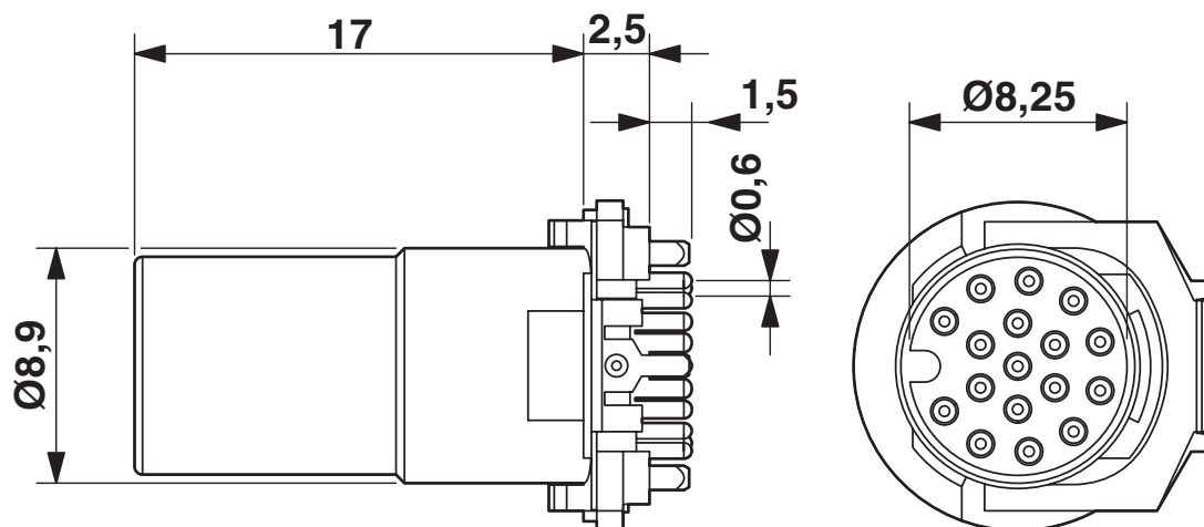
Rysunek wymiarowy
