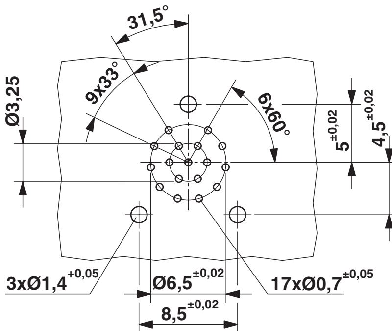
Otworowanie/geometria płytek lutowniczych
