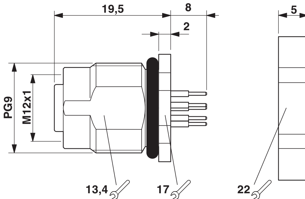
Rysunek wymiarowy
