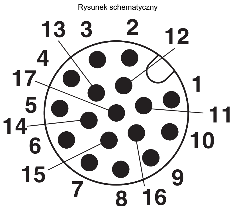
Układ styków, wtyk M12, 17-biegunowy, widok od strony styków
