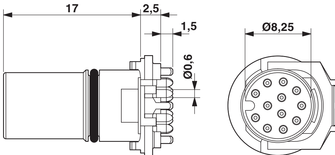
Rysunek wymiarowy
