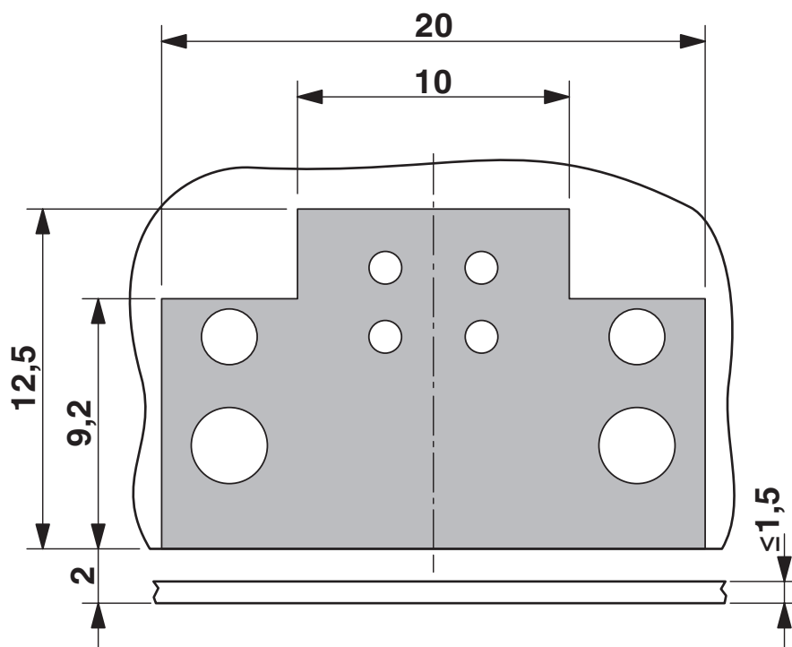
Rysunek wymiarowy
