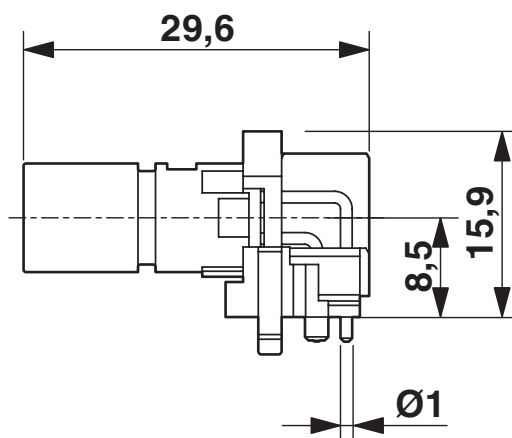
Rysunek wymiarowy
