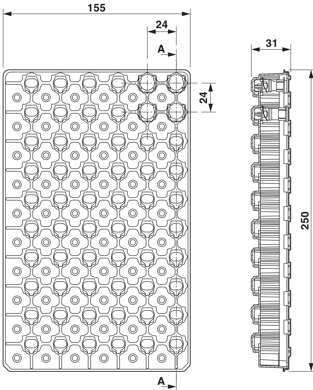
Rysunek wymiarowy
