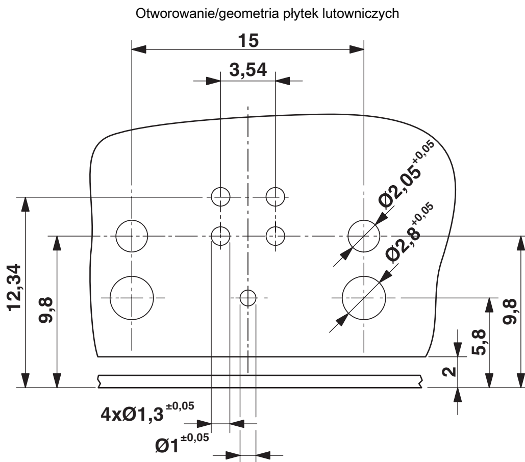
Rysunek wymiarowy
