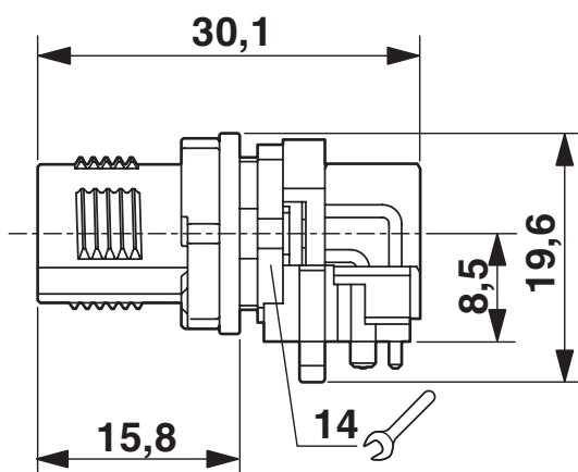
Rysunek wymiarowy
