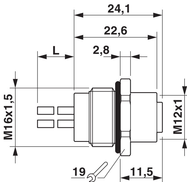
Rysunek wymiarowy
