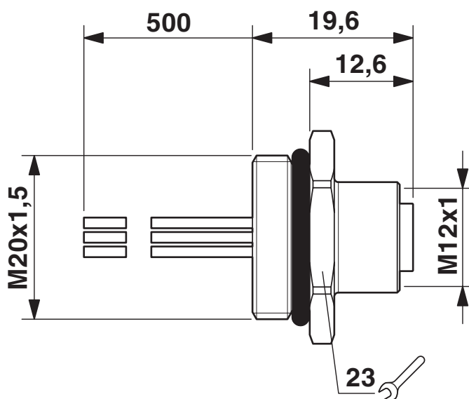
Rysunek wymiarowy
