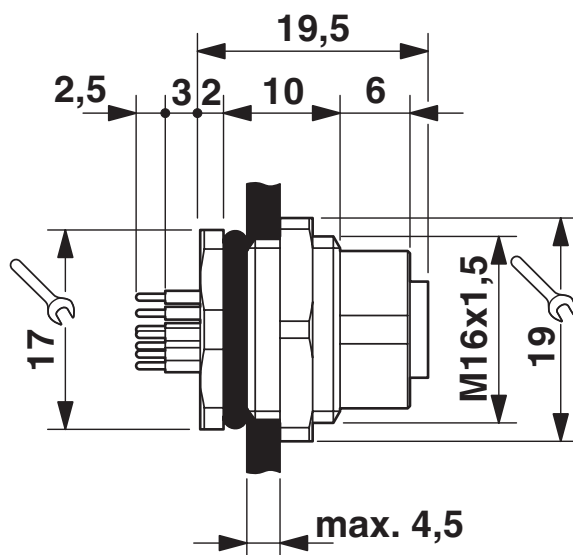
Rysunek wymiarowy
