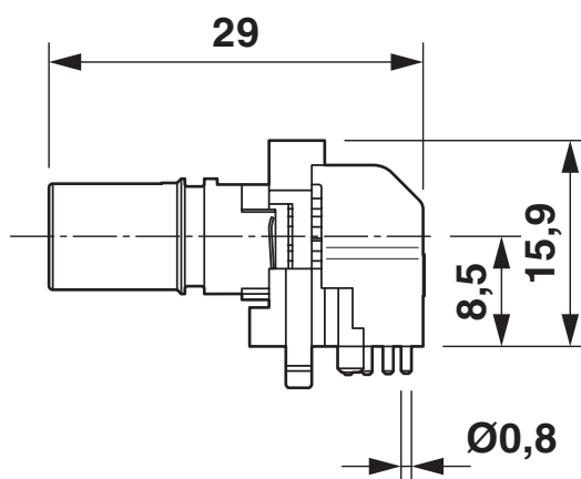
Rysunek wymiarowy
