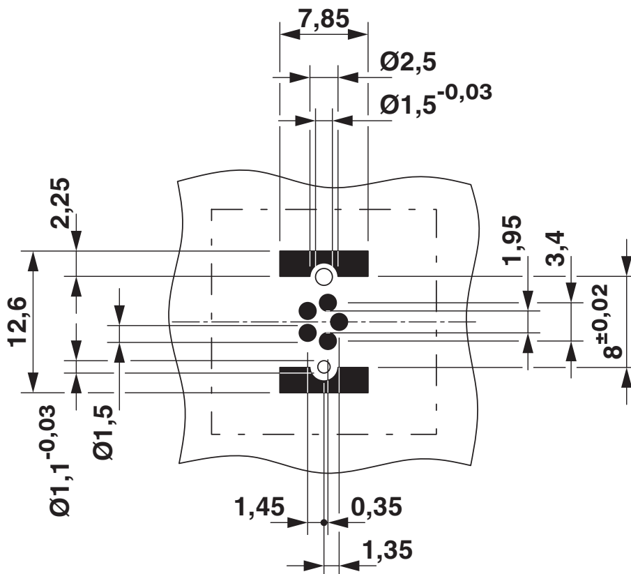
Otworowanie/geometria płytek lutowniczych
