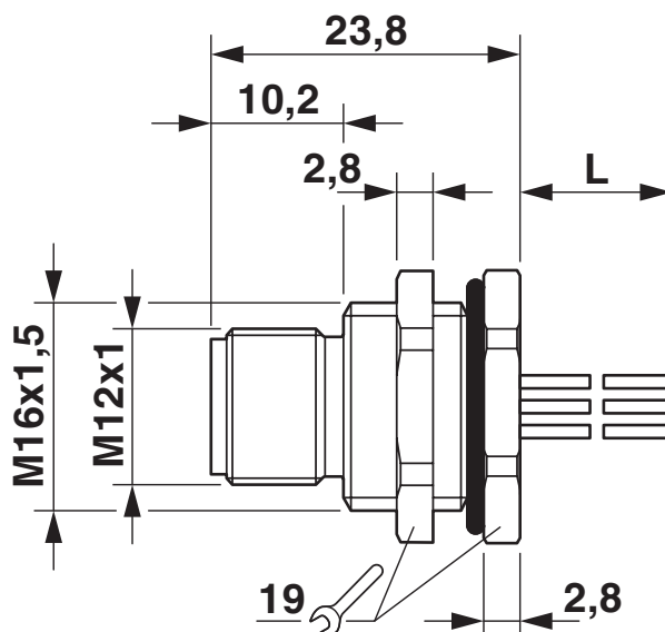
Rysunek wymiarowy
