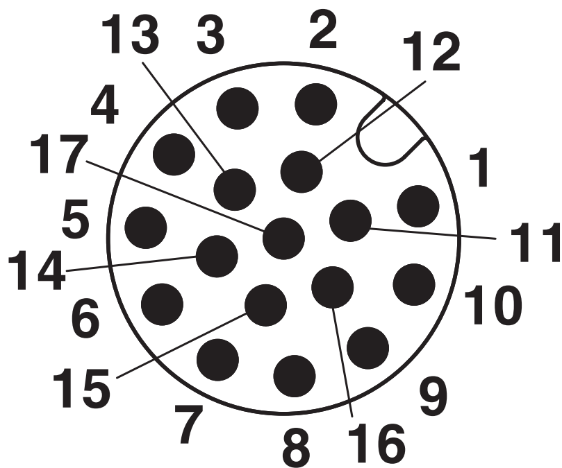
Rysunek schematyczny
