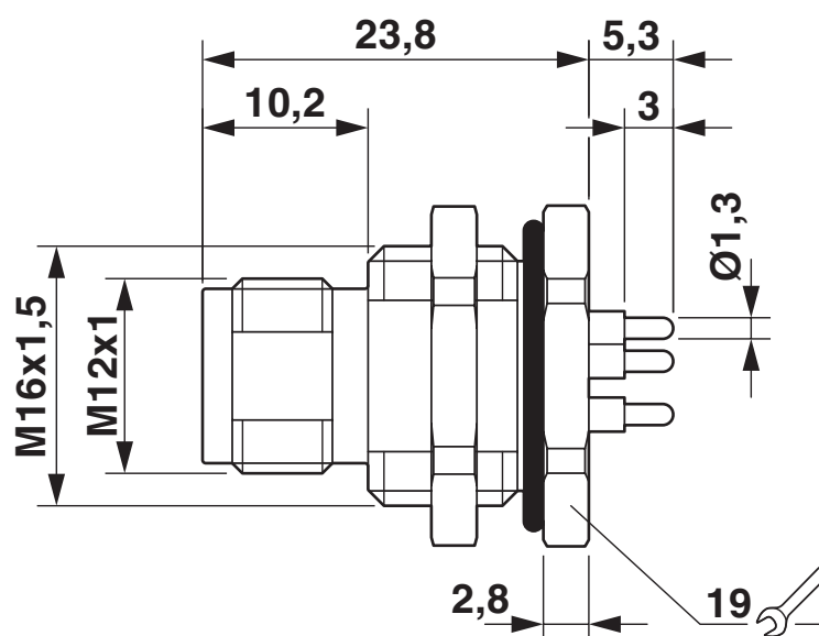
Rysunek wymiarowy
