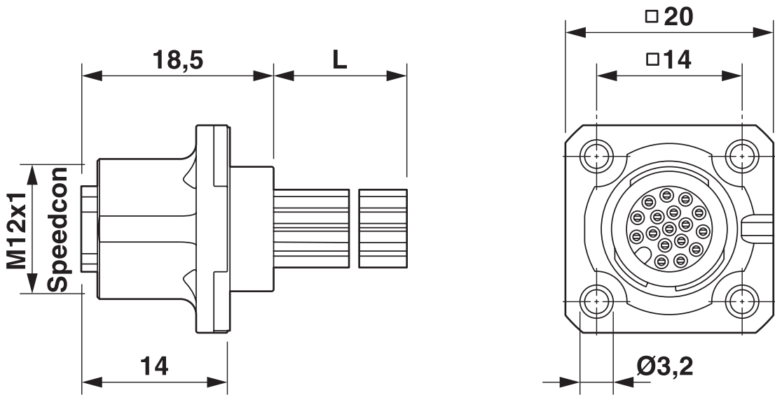
Rysunek wymiarowy
