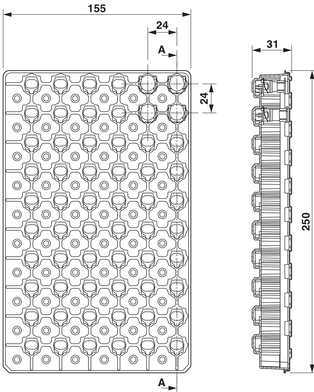
Rysunek wymiarowy
