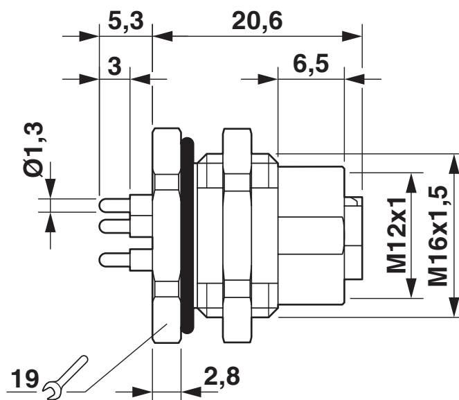
Rysunek wymiarowy
