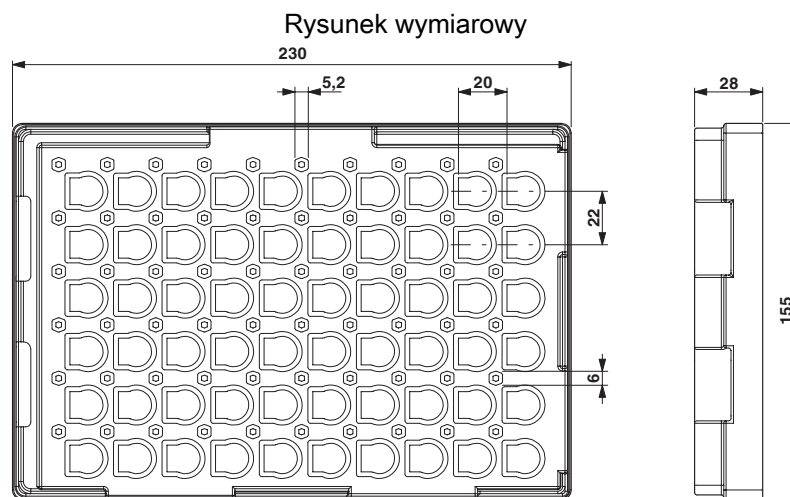
Rysunek schematyczny
