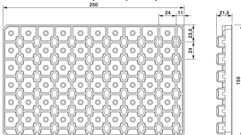
Rysunek wymiarowy
