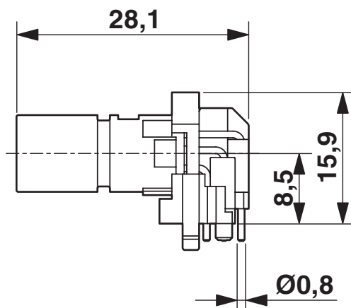
Rysunek wymiarowy
