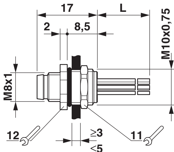
Rysunek wymiarowy
