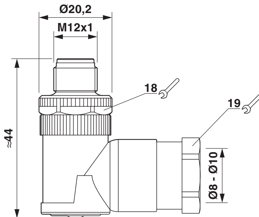
Rysunek wymiarowy
