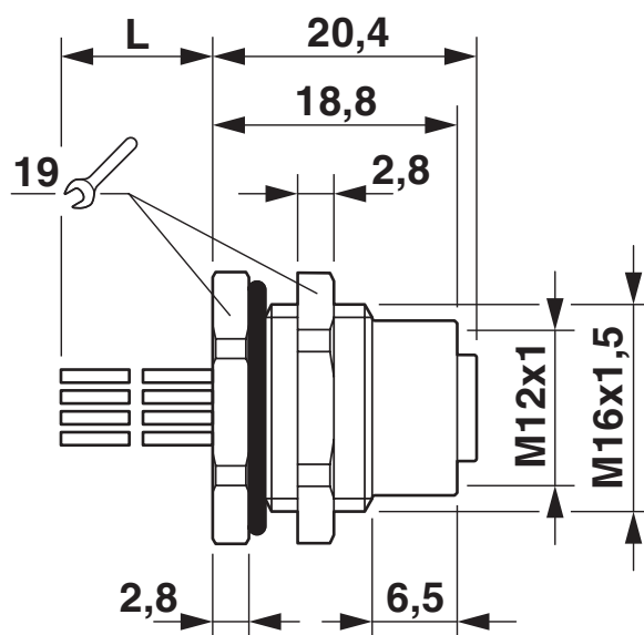
Rysunek wymiarowy
