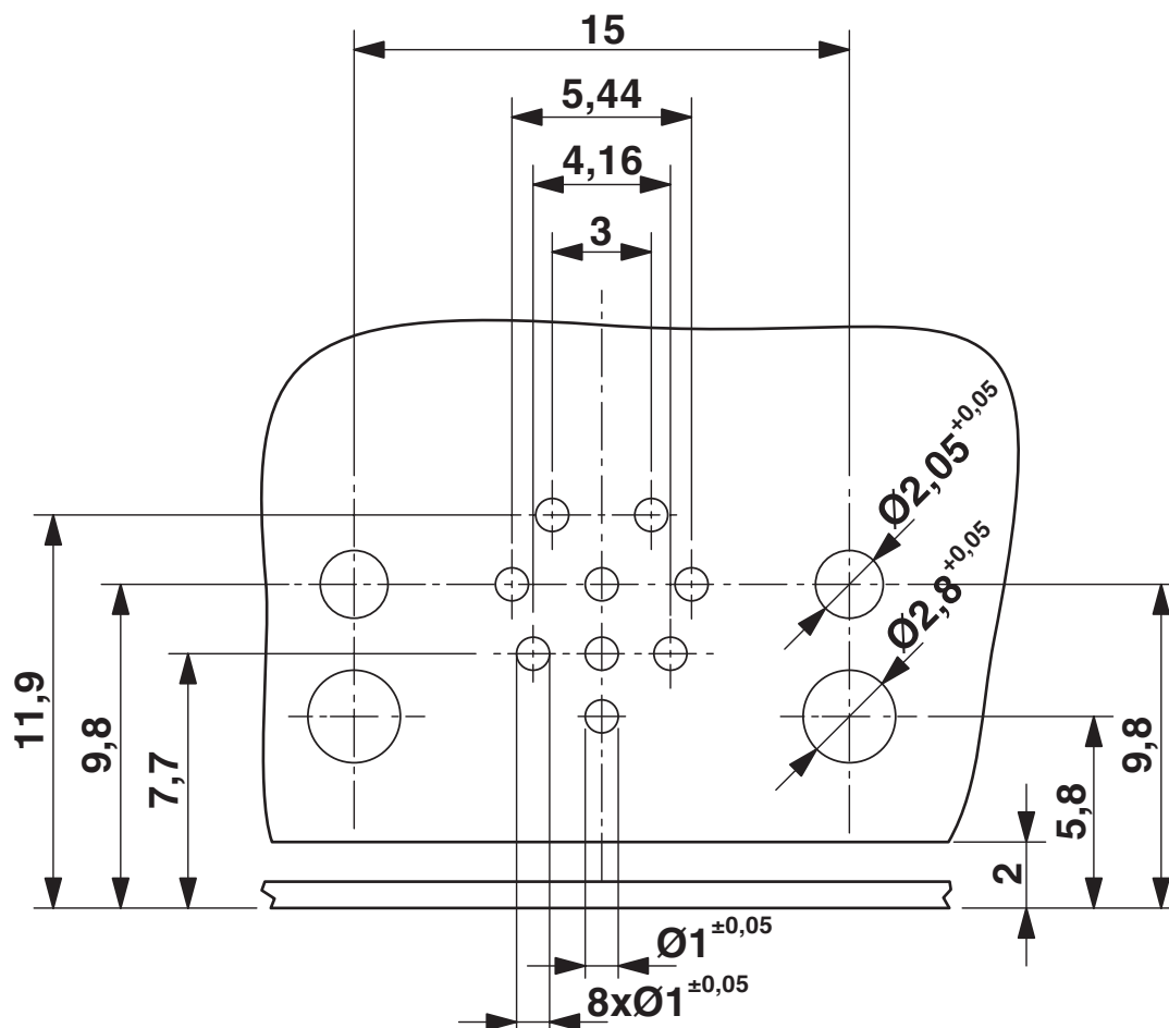
Otworowanie/geometria płytek lutowniczych
