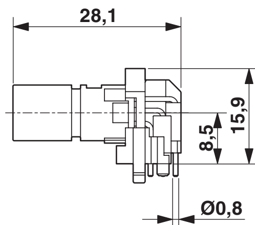
Rysunek wymiarowy
