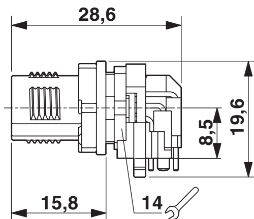
Rysunek wymiarowy
