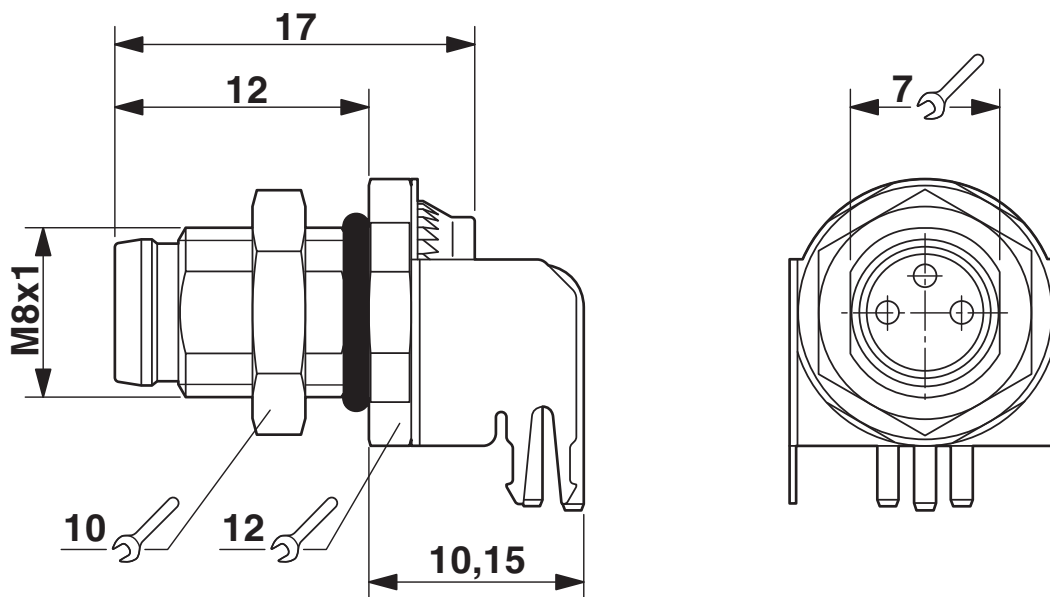
Rysunek wymiarowy
