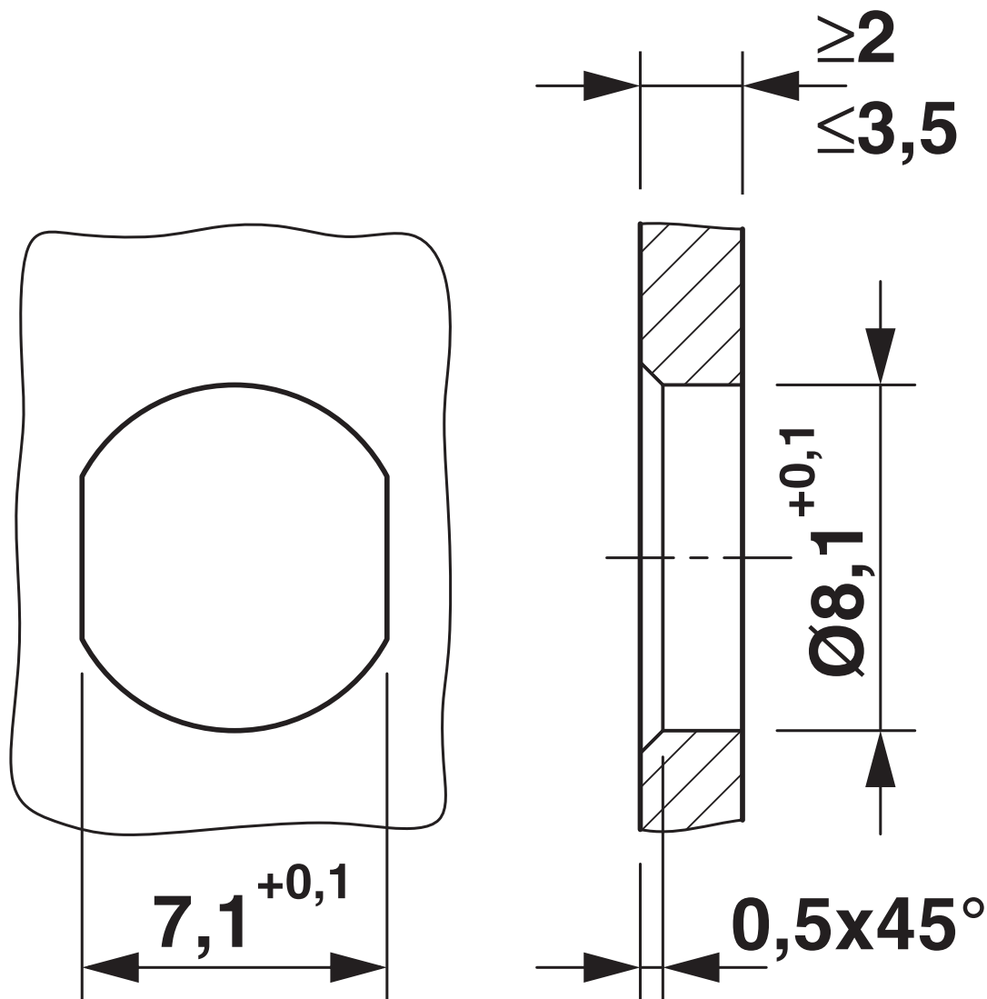
Rysunek wymiarowy
