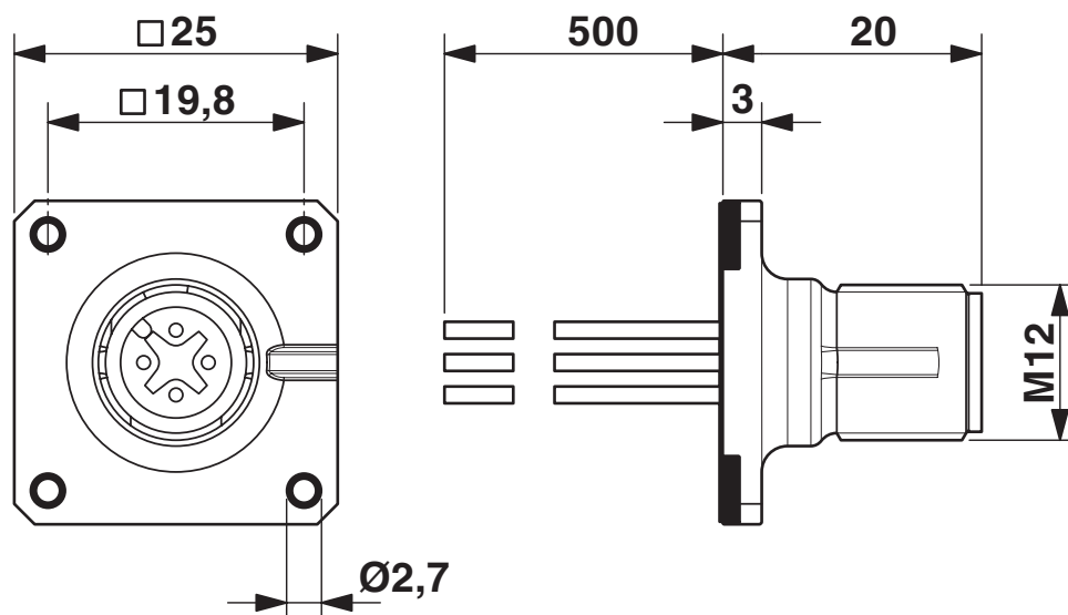
Rysunek wymiarowy
