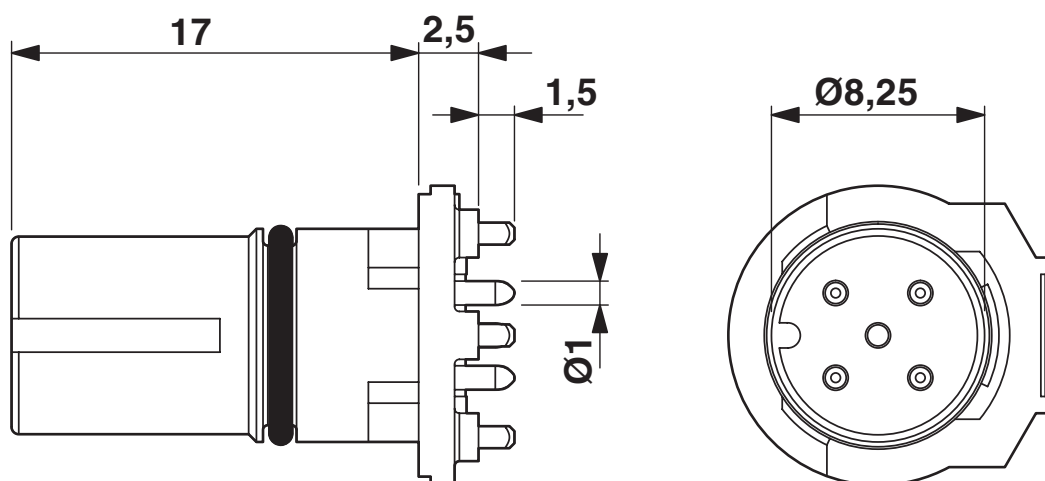
Rysunek wymiarowy
