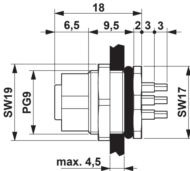
Rysunek wymiarowy
