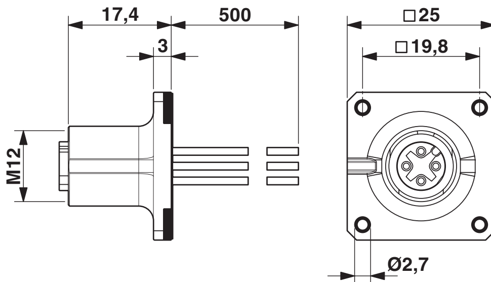
Rysunek wymiarowy
