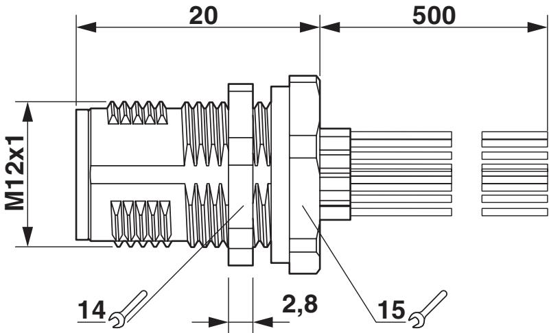
Rysunek wymiarowy
