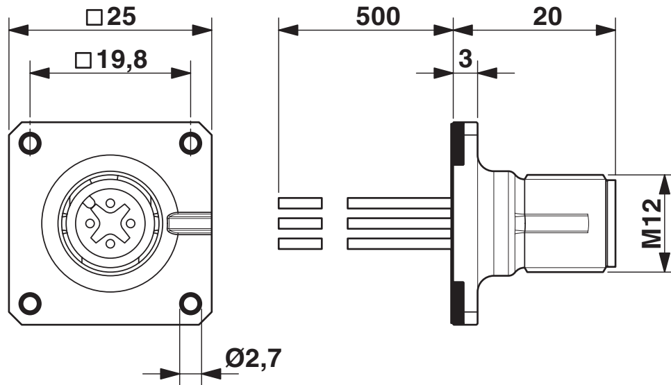
Rysunek wymiarowy
