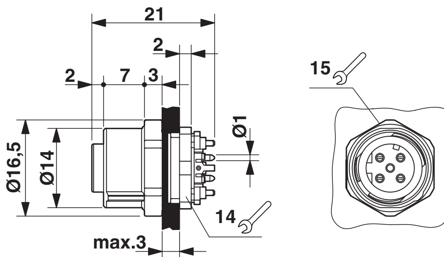
Rysunek wymiarowy
