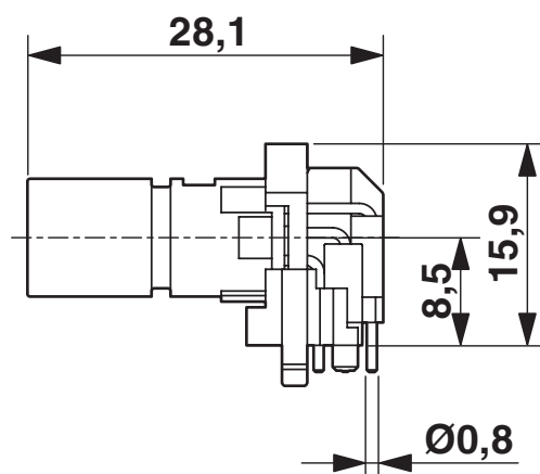
Rysunek wymiarowy
