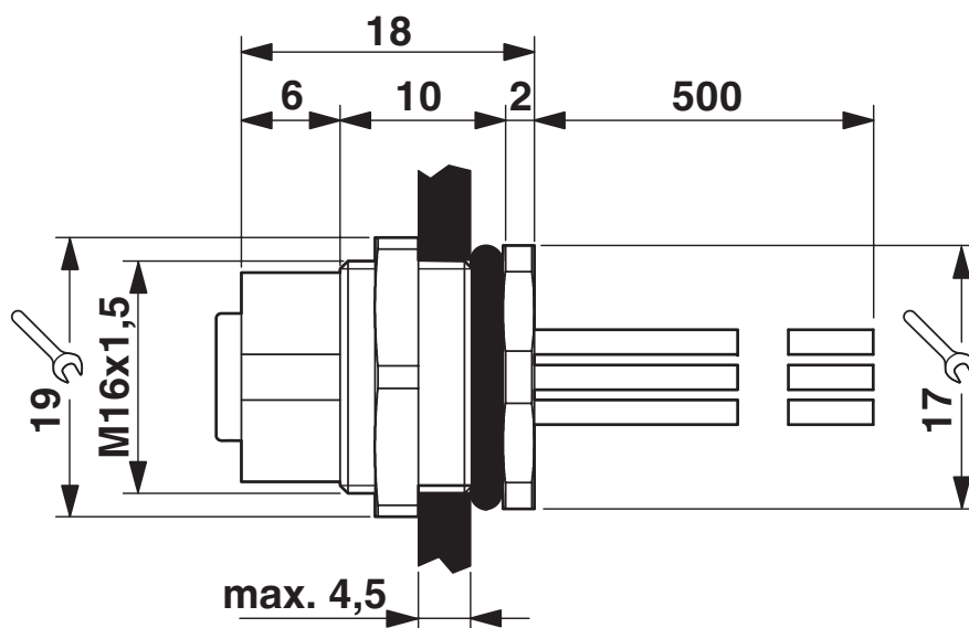
Rysunek wymiarowy
