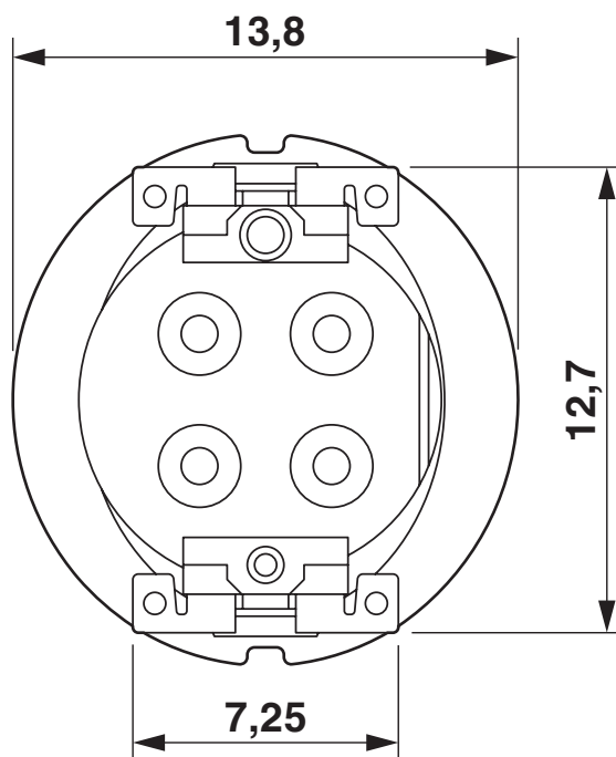
Rysunek wymiarowy
