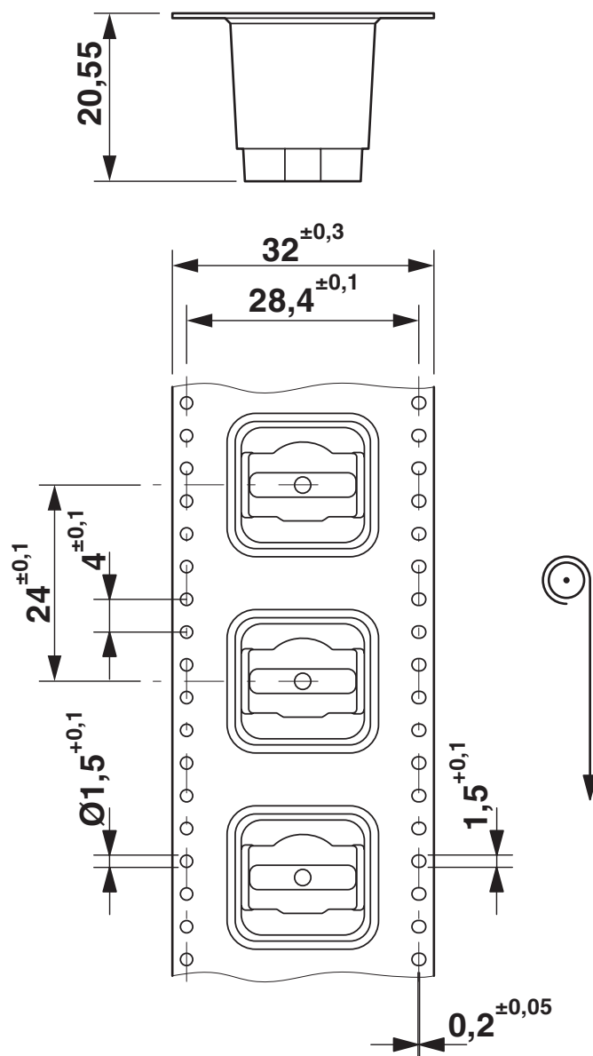
Rysunek wymiarowy
