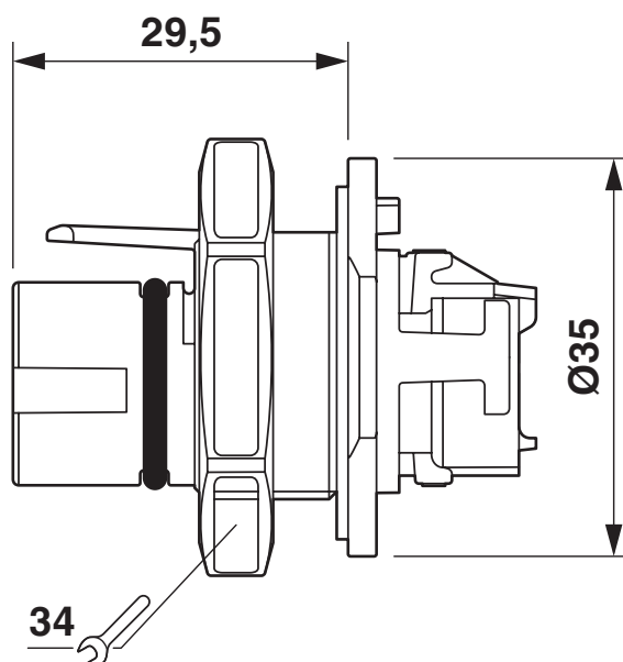
Rysunek wymiarowy
