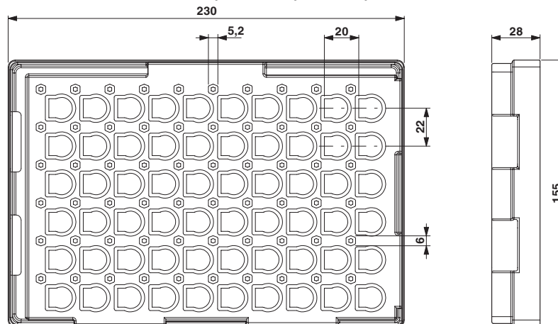
Rysunek wymiarowy
