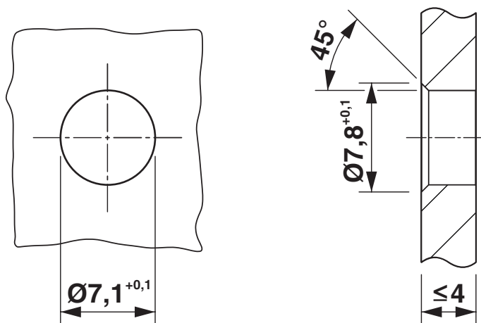
Rysunek wymiarowy
