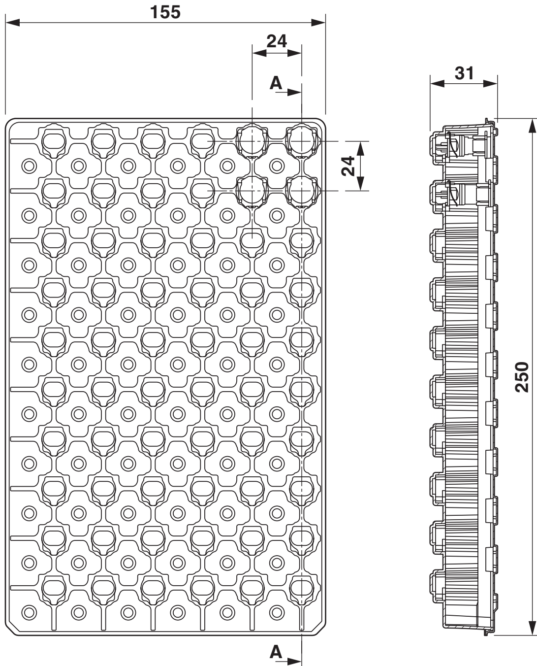
Rysunek wymiarowy
